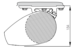
Deckenmontage Jubilo
